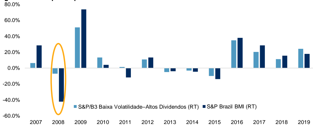
Figura 3: Desempenho por ano-calendário
