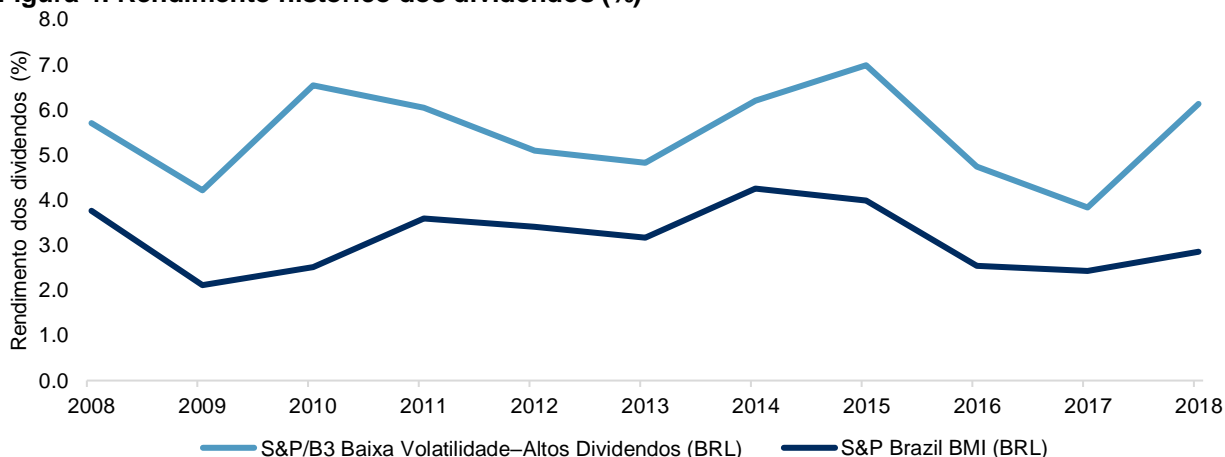
Figura 4: Rendimento histórico dos dividendos (%)
