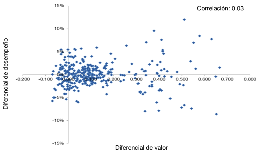
Figura 1: El gráfico de dispersión de las puntuaciones de valor relativo mensual y diferencial de desempeño del S&P 500 Low Volatility Index al mes siguiente no muestra una relación
